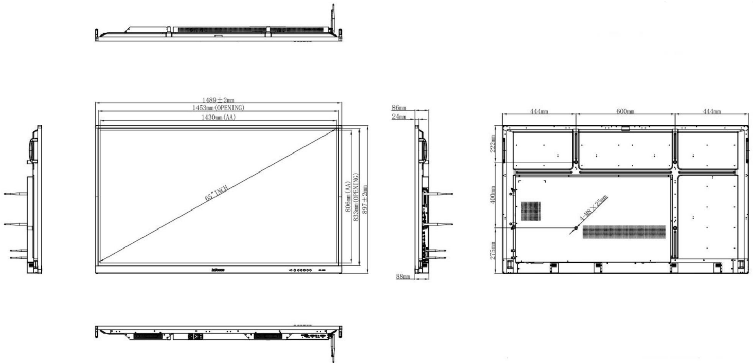
DGTK65FA
